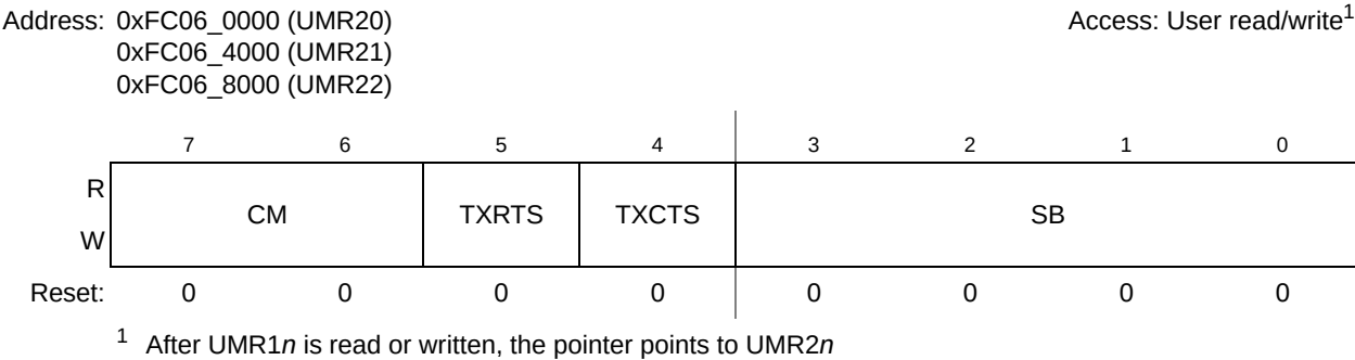
Figure 31-4. UART Mode Registers 2 (UMR2n)
